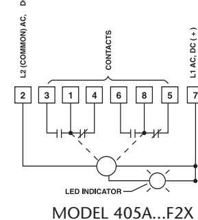
WIRING
