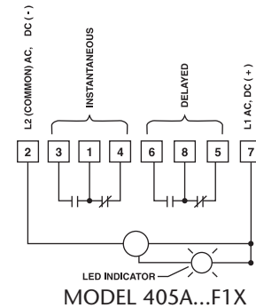
WIRING
